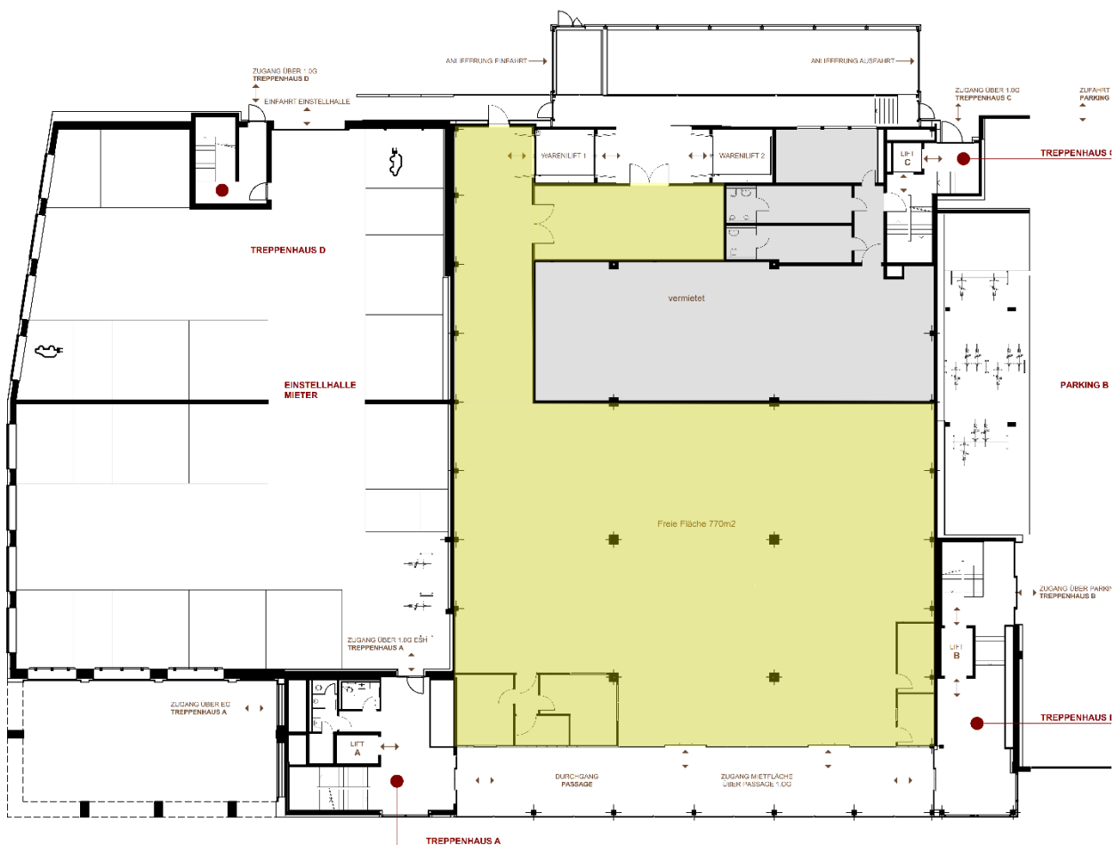
Grundriss: erstes Obergeschoss, 770 m 2 Nutzfläche
